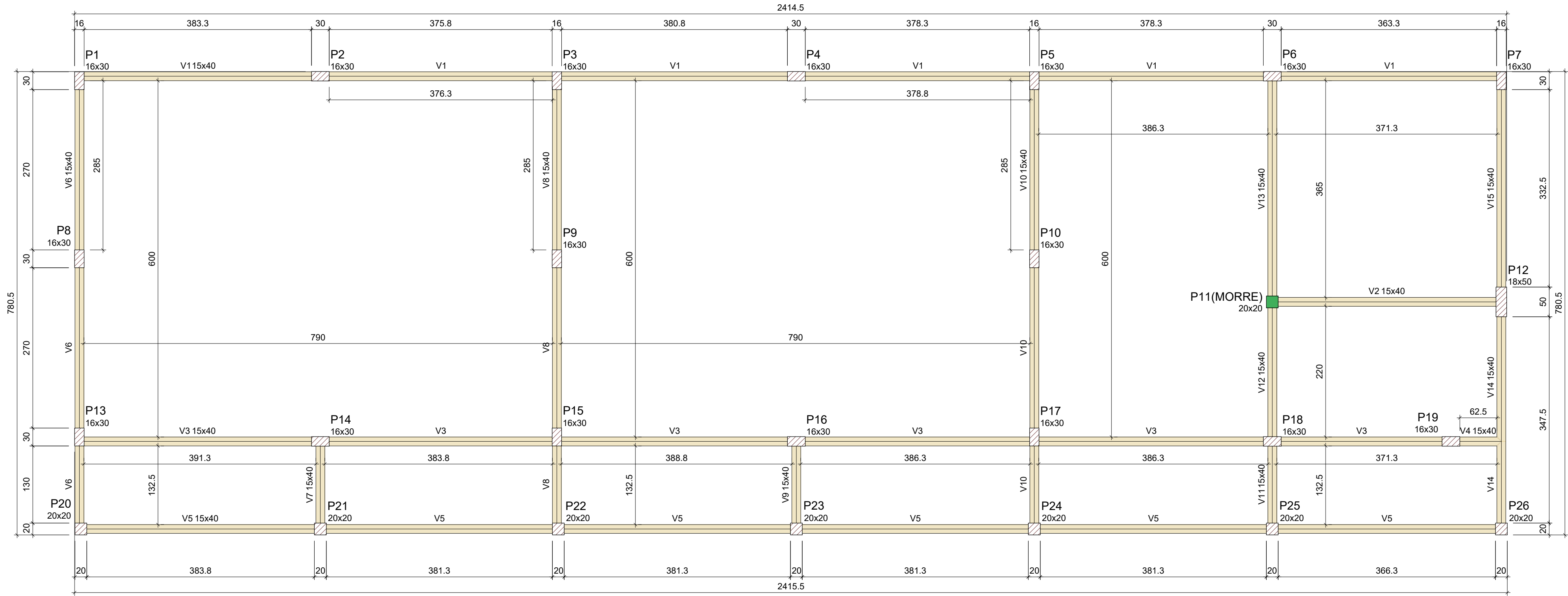
1 PLANTA DE FÔRMAS BALDRÂME - PEDAGÓGICO ESCALA 1/50
